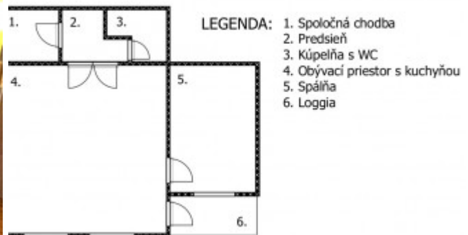
Pôdorys 2-izbového bytu
